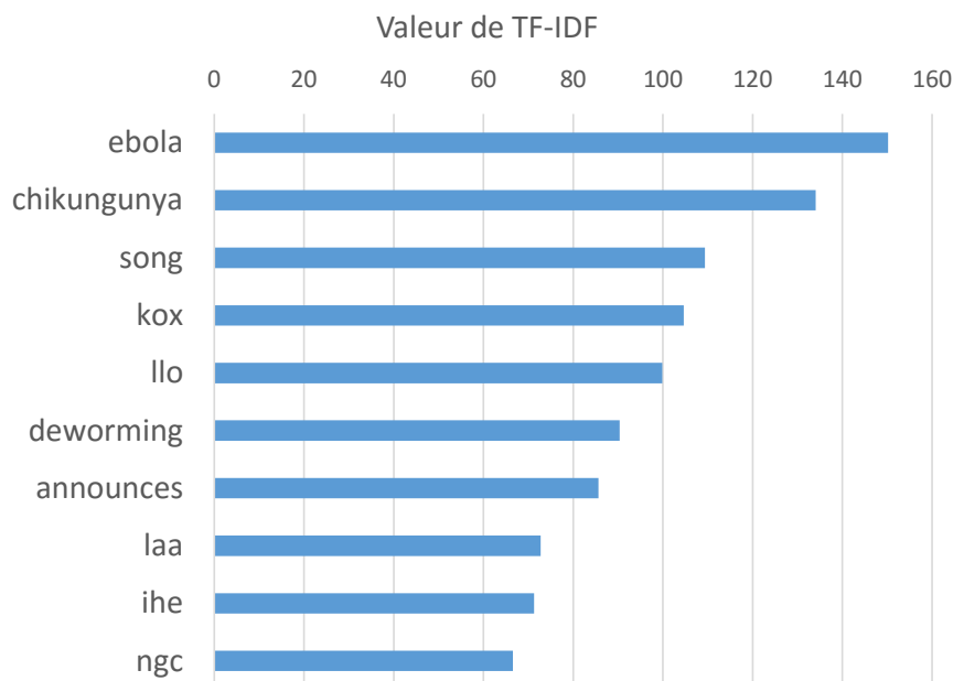
FIGURE 5.8. Liste des mots du corpus ayant les grandes valeurs de pondération tf-idf . On remarque que les mots clés du cluster signal faible détecté sont parmi les premiers de la liste.
