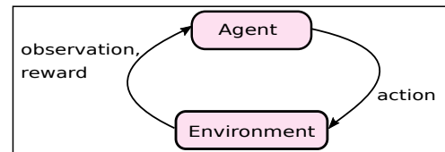
Fig. 3. MDP model.
