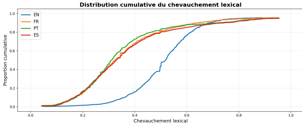
FIGURE 1 – Distribution cumulative du chevauchement lexical moyen requêtes-documents
